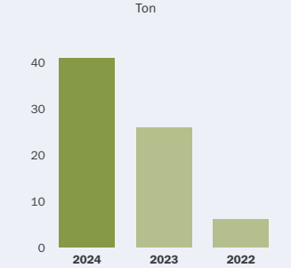
305-3 Övriga indirekta utsläpp av växthusgaser (scope 3), intern
