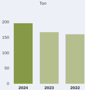
305-2 Indirekta utsläpp av växthusgaser (scope 2), extern
