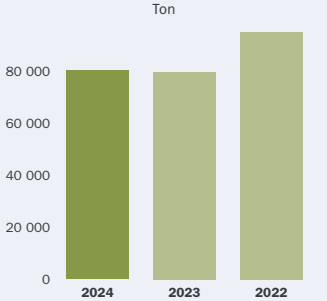
305-3 Övriga indirekta utsläpp av växthusgaser (scope 3), extern
