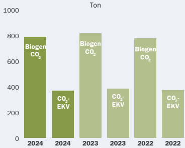
305-2 Indirekta utsläpp av växthusgaser (scope 2), intern
