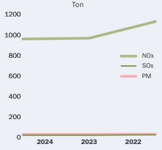
305-7 Emissioner, fartyg inom hamnområden
